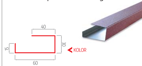
listwa podgąsiorowa do panelu dachowego
