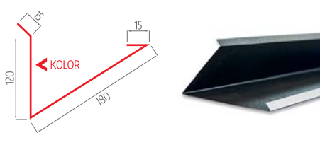
obróbka kominowa górna standard Z 33 cm
