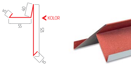
wiatrownica standard Z 25 cm
