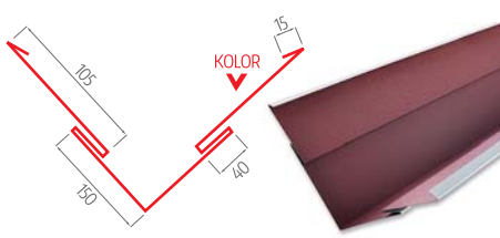
kosz do panelu dachowego Z 62 cm
