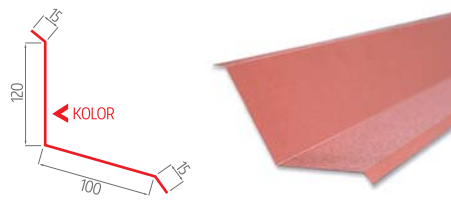
obróbka obok ściany i kominowa boczna standard Z 25 cm na blachę
