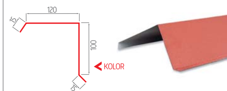
wiatrownica standard Z 25 cm na blachę
