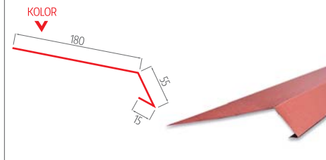
pas nadrynnowy standard Z 25 cm
